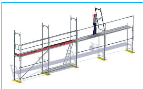
Art.no. 4030/307 Garde-corps de montage T19, réglable.
