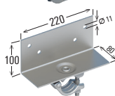
Collier grand avec cornière pour raccord d'éléments bois/acier carrés Art.no. : 4717/019 / 4717/022
