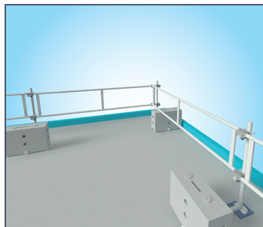
Compacte plat dakrandbeveiliging gemonteerd met rolsteigerleuning.
