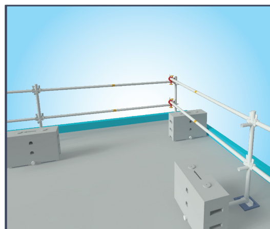
Compacte plat dakrandbeveiliging gemonteerd met Allroundliggers.
