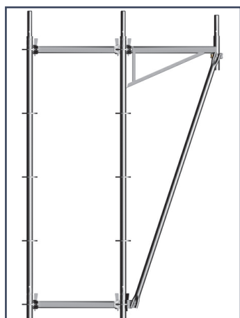
Console 0.73 m. avec support.
