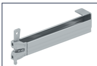
2618/038 Lisse de console avec 1 tête de clavette, application en U.
