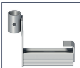
2632/001 Extension pour console Allround, application en U.
