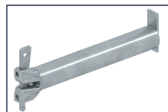
0735/743 Lisse de console avec 1 tête de clavette, application en tube.
