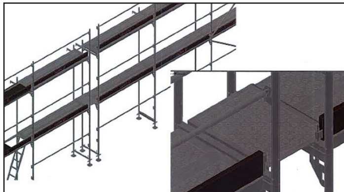
Planchers d'étanchéité zones de compensations no.d'article 3868.061
